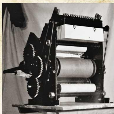
Podziemna myśl techniczna – „Łakomiec”, powielacz offsetowy opracowany i wykonany przez Wydawnictwo Myśli Nieinternowej z Krakowa.
